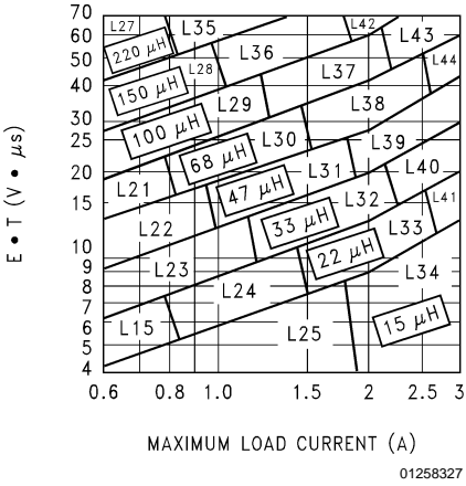
FIGURE7.LM2596/LM2596HV-ADJ
