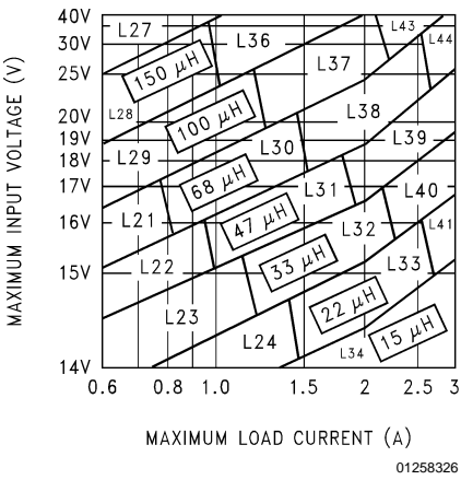
FIGURE6.LM2596/LM2596HV-12
