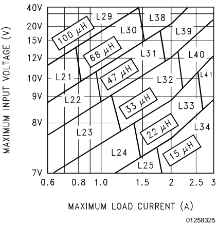
FIGURE5.LM2596/LM2596HV-5.0
