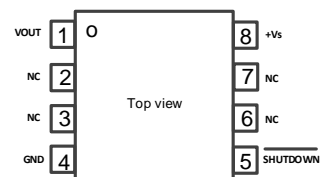
Figure4. SOIC
